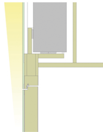
Detail Glaswand mit flächenbündig integrierter Tür Detail of integrated door flush with glass covered wall
